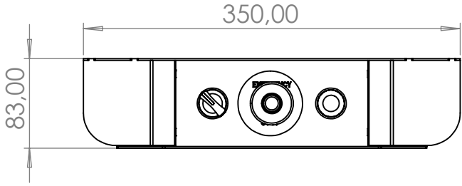
ÜST GÖRÜNÜS
