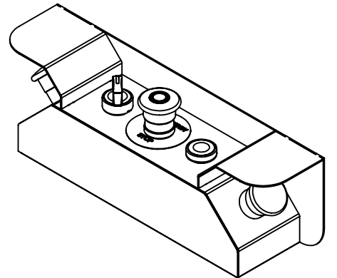
TRİMETRİK GÖRÜNÜS
