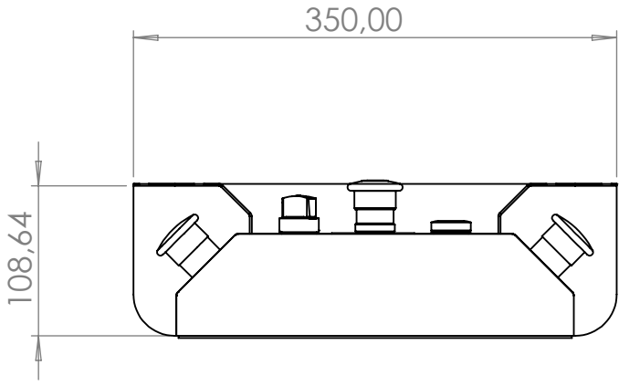
KARŞIDAN GÖRÜNÜS
