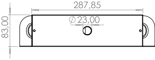
ALT GÖRÜNÜS
